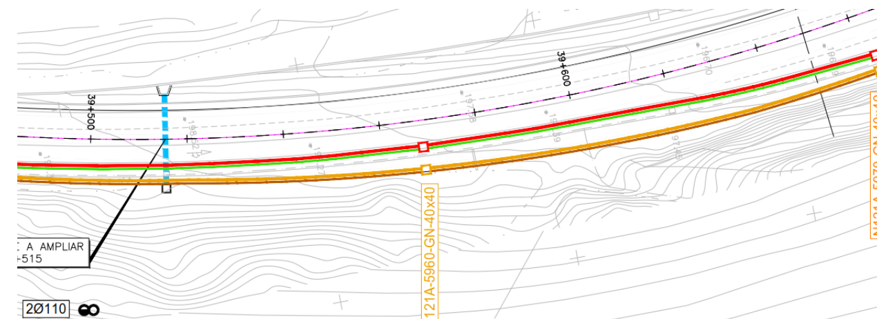
Imagen 7: Representación de un tramo de la zona de estudio (PK 39+600), donde se aprecia la separación entre la canalización actual (rojo) y la proyectada (naranja).
