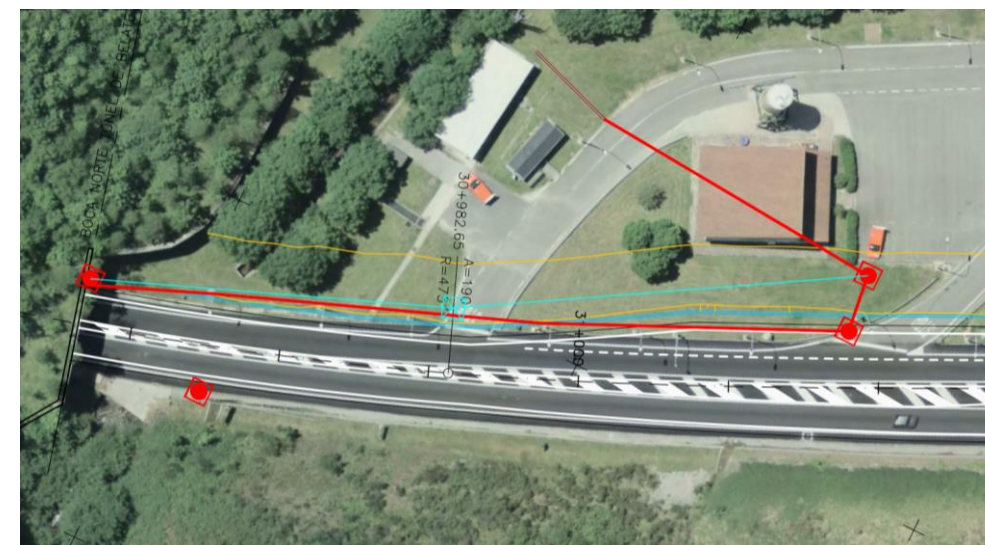
Imagen 4- Reposición proyectada para la afección a canalización telefónica existente a la salida del túnel de Belate (PK 31+000)
