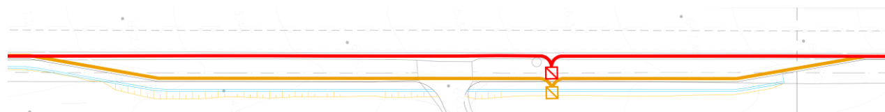
Imagen 2: (Superior) Fotografía de la zona reflejada, indicando en la imagen la situación de la arqueta. (Inferior) Representación del tramo, donde se aprecia el desplazamiento de la red de fibra óptica proyectada (naranja) respecto a la original (rojo).
