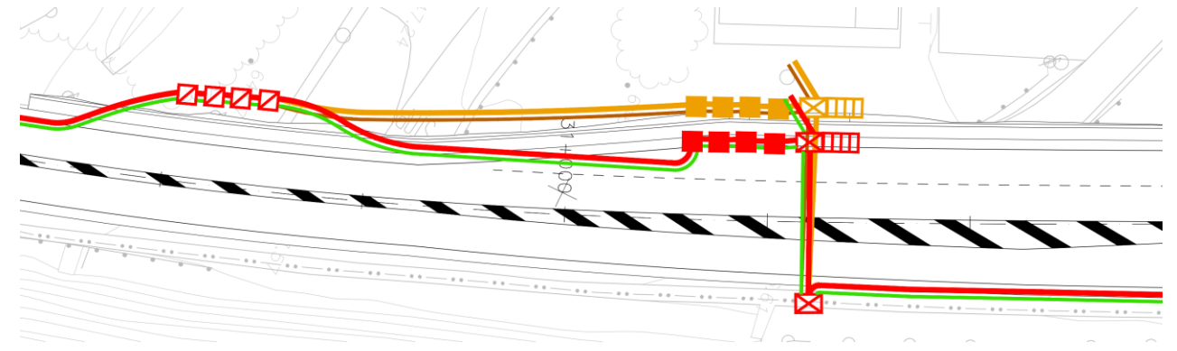
Imagen 3: (Superior) Fotografía de la zona reflejada (Inferior) Representación del tramo, donde se aprecia el desplazamiento de la red de fibra óptica proyectada (naranja) respecto a la original (rojo).
