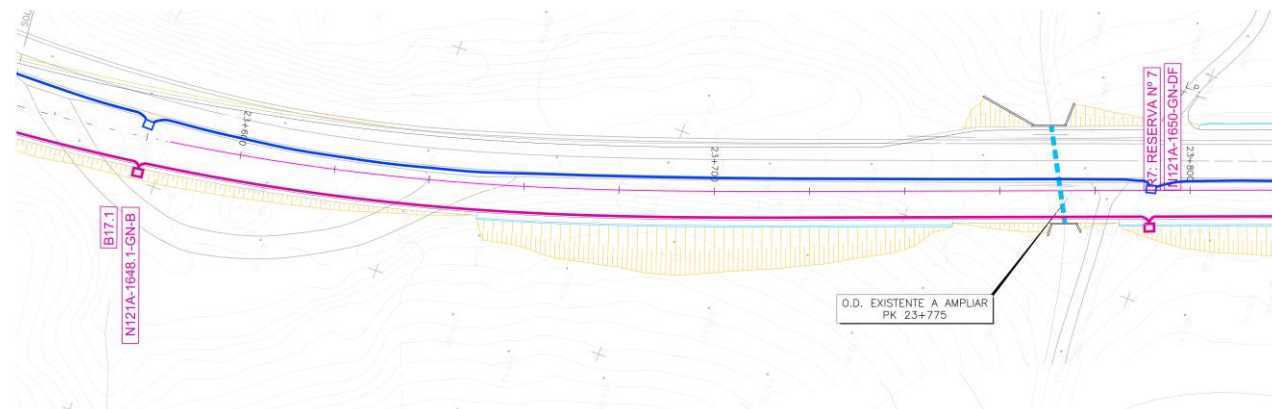
Imagen 1: Representación de un tramo de la zona de estudio (PK 23+700), donde se aprecia la separación entre la canalización actual (azul) y la proyectada (magenta).
