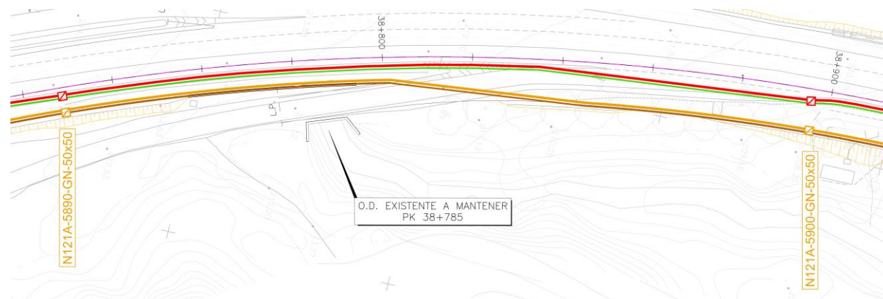
Imagen 6: Representación de un tramo de la zona de estudio (PK 38+800), donde se aprecia la separación entre la canalización actual (rojo) y la proyectada (naranja).
