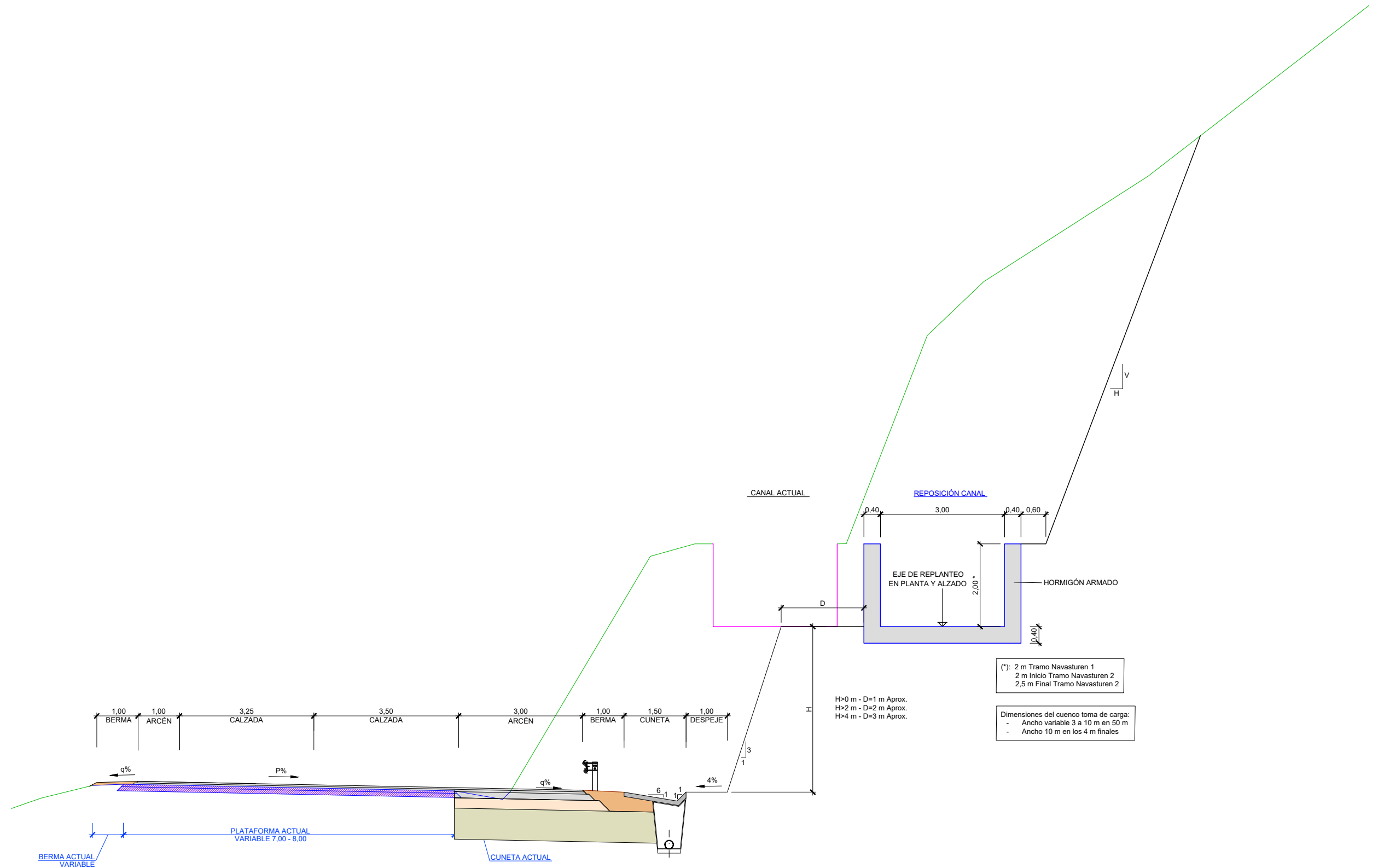
SECCIÓN CANAL NAVASTUREN JUNTO A CALZADA DERECHA SOBRE NA-1210 ESCALA 1:100
