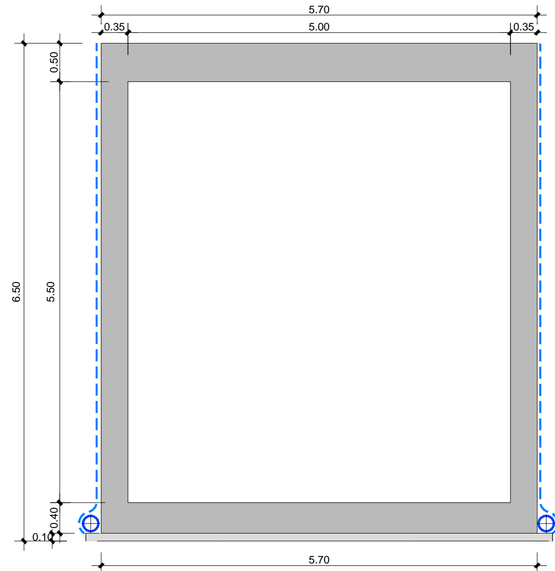
SECCIÓN TRANSVERSAL MARCO DEFINICIÓN GEOMÉTRICA ESCALA 1/50
