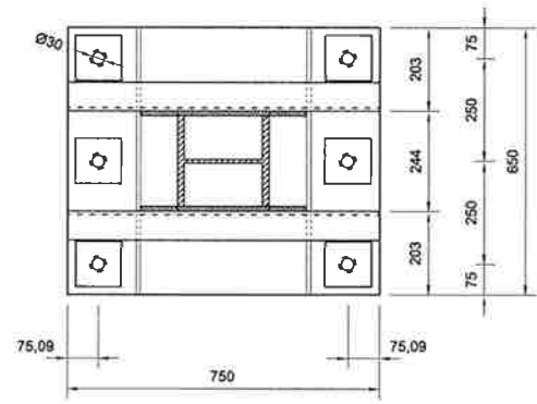
DETALLE 6
