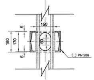
DETALLE 7
